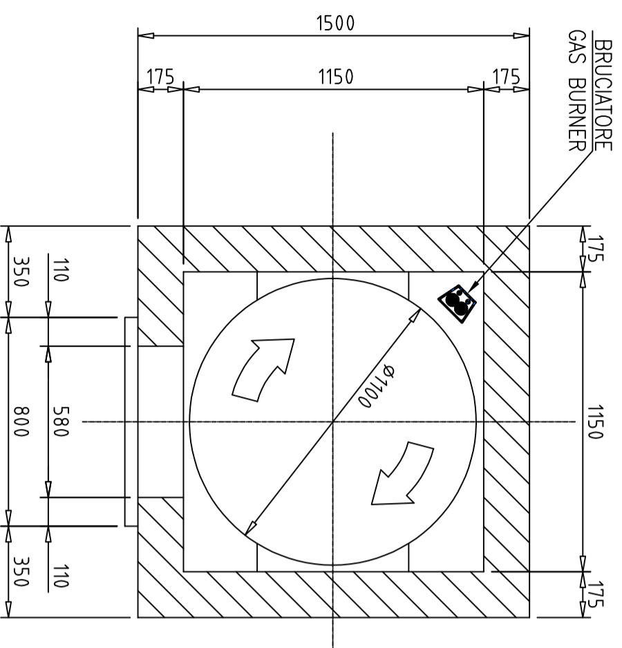
VISTA SEZIONATA IN PIANTA
