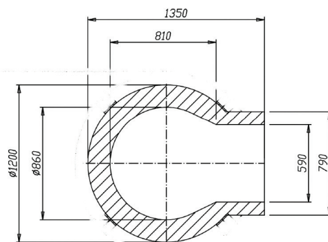
SEZIONE IN PIANTA INTERNO FORNO
