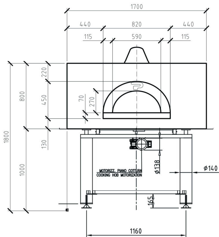
Vista sezionata in pianta
